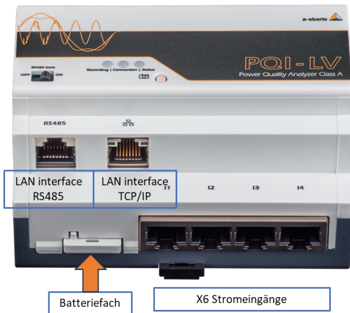
Seitenansicht PQI-LV
