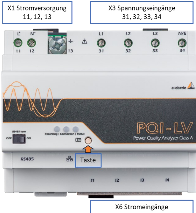
Frontansicht PQI-LV
